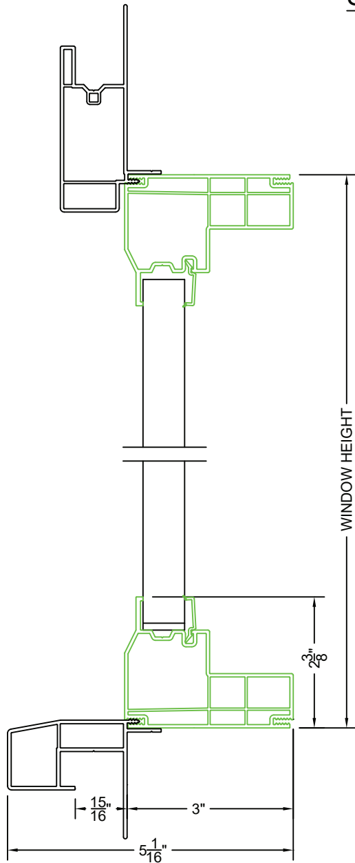
SECTION A-A SCALE: 1:1
